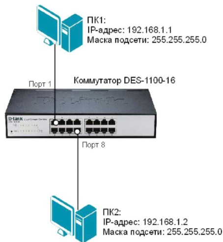
Рисунок 1 - Схема подключения типа «компьютер-
