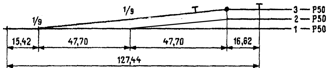
Рисунок 8 Образец выполнения стрелочной улицы по основному пути в масштабе 1:2000
