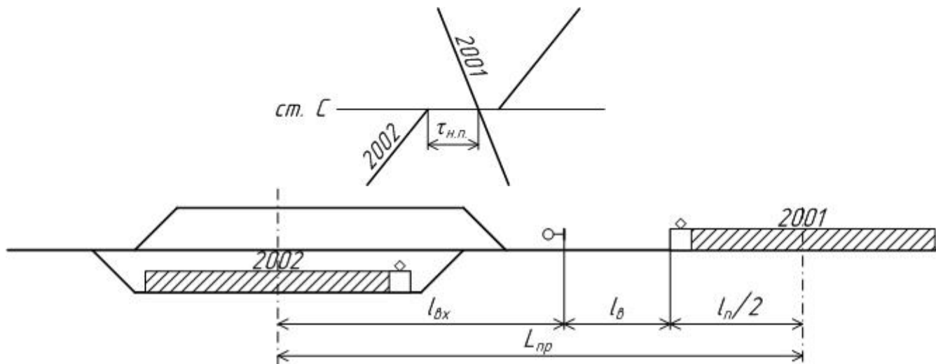
Рисунок 3 Схема расположения поездов при расчете интервала неодновременного прибытия при полуавтоматической блокировке
