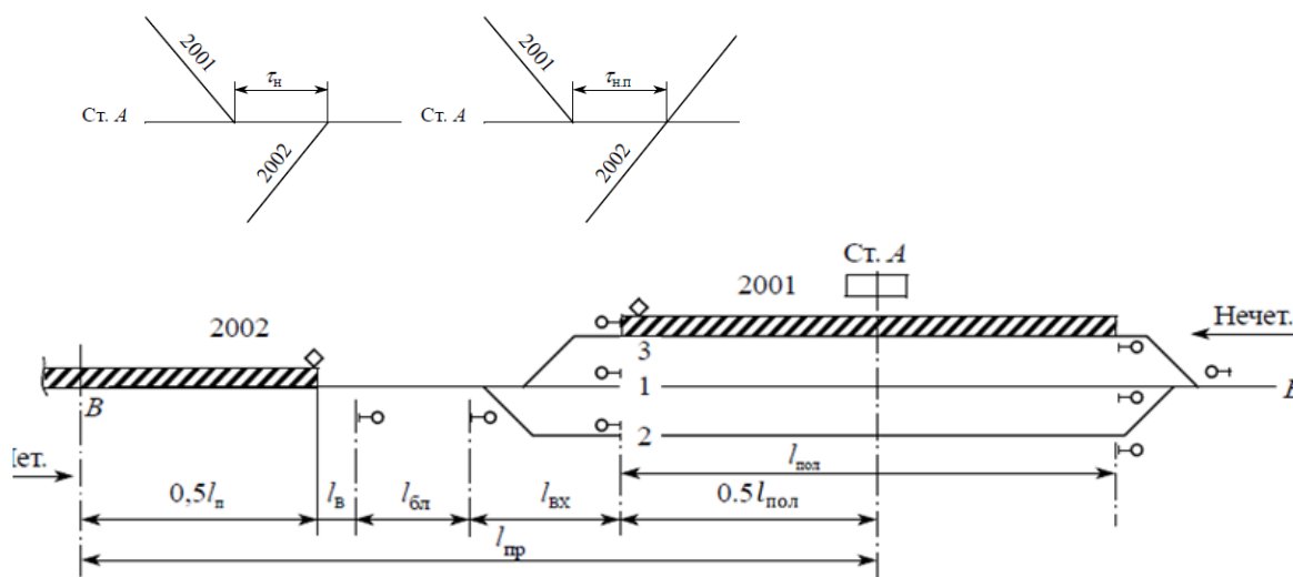
Рисунок 1 Схема расположения поездов при расчете интервала неодновременного прибытия при автоматической блокировке
