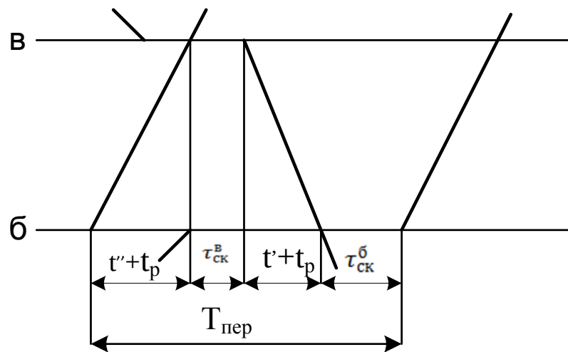
Схема 2 - поезда следуют с труднейшего перегона сходу;
