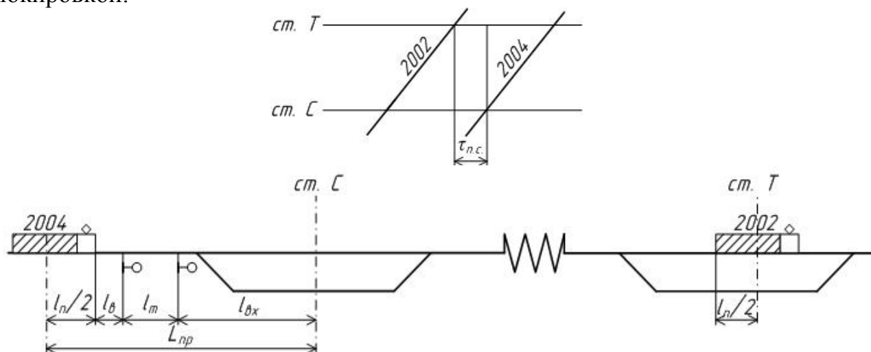
Рисунок 8 Схема расположения поездов при расчете интервала попутного следования при полуавтоматической блокировке
