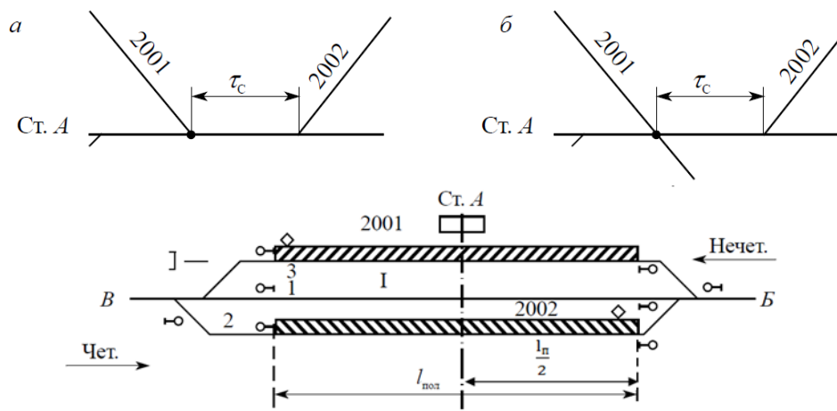
Рисунок 5 Схема расположения поездов при расчете интервала скрещения
