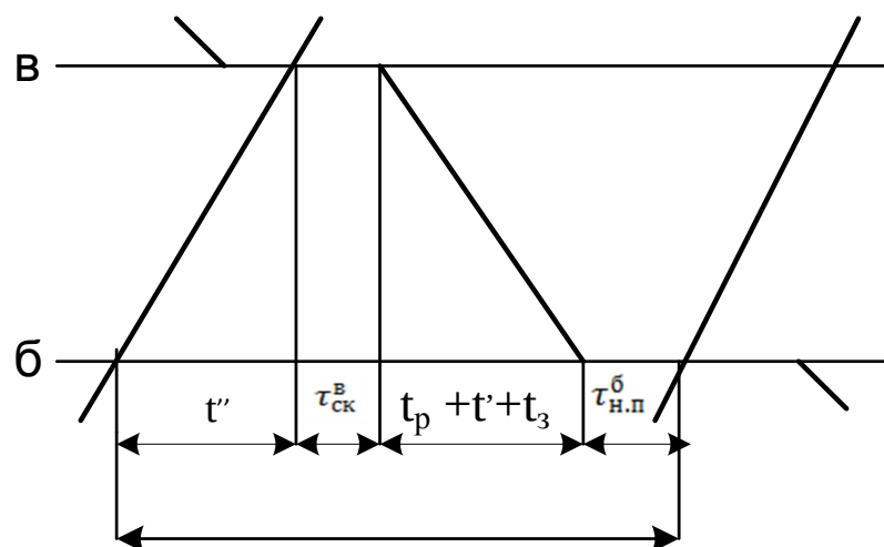
Схема 4 - четные поезда следуют по труднейшему перегону сходу.
