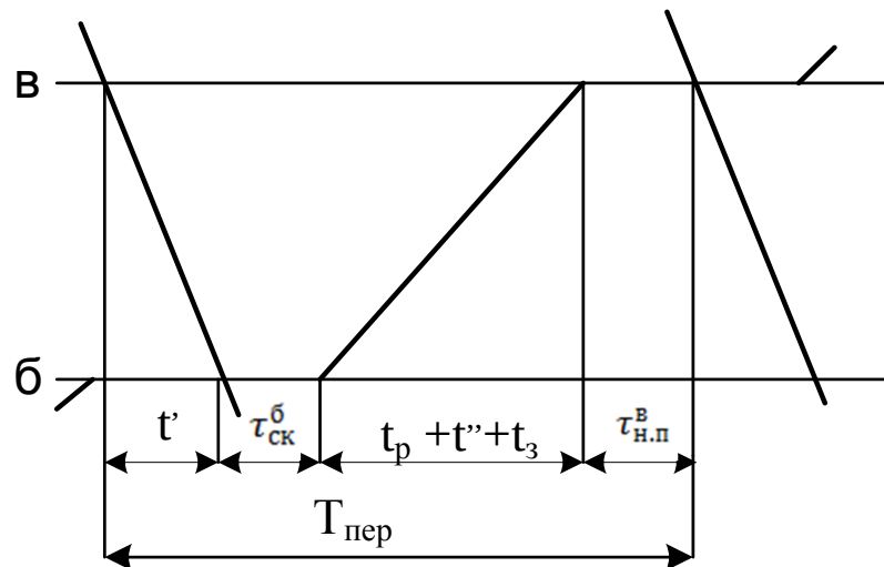
Схема 2 - поезда следуют с труднейшего перегона сходу;
