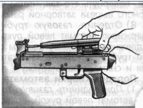
Рис. 6. Отделение затворной рамы с затвором
