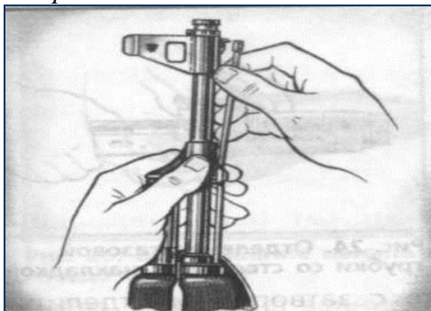
Рис 9. Присоединение шомпола
