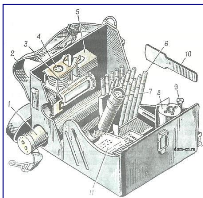
Рис. 7. Войсковой прибор химической разведки (ВПХР): 1 - ручной насос; 2 - плечевой ремень с тесьмой; 3 - насадка к насосу; 4 - защитные колпачки для насадки; 5 - противодымные фильтры; 6- патрон грелки; 7 - электрический фонарь; 8 - корпус грелки; 9 - штырь; 10 - лопатка; 11 - индикаторные трубки в кассетах
