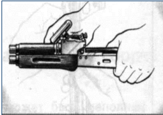
Рис. 8. Отделение газовой трубки со ствольной накладкой
