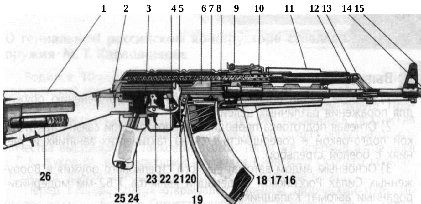
Рис. 1. 7,62-мм АКМ:
