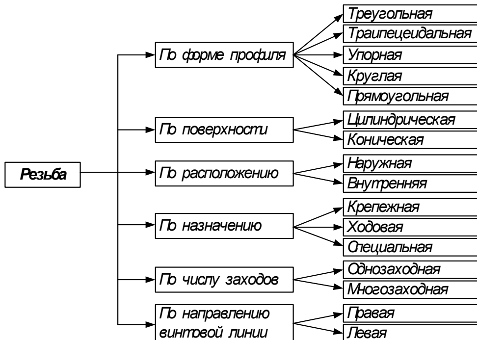
Рисунок 1 Классификация резьбы
