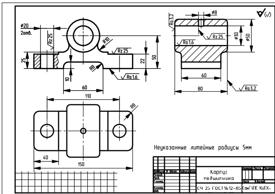
Рисунок 10 Эскиз детали
