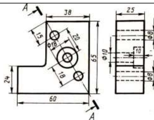
Стойка
