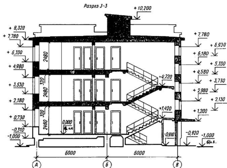
Рисунок 5 Порядок построения чертежа разреза здания
