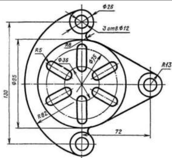
Решетка
