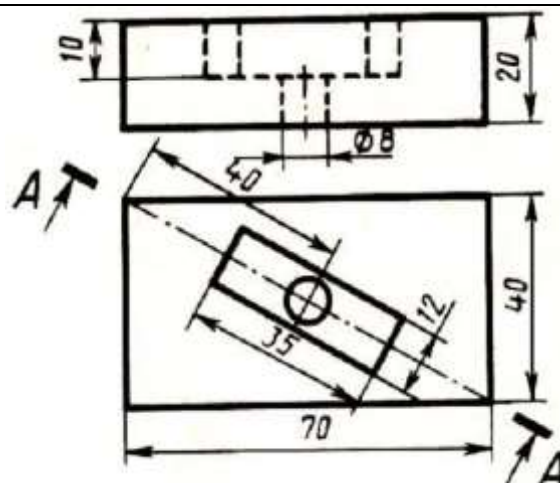
Плита
