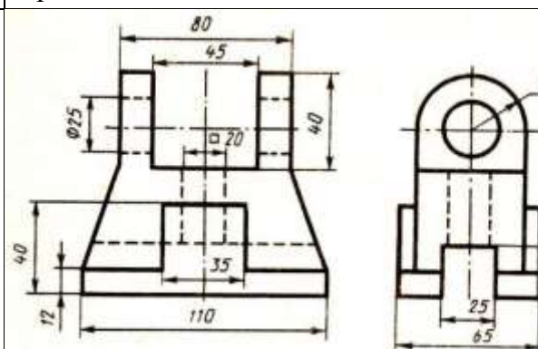
Кронштейн
