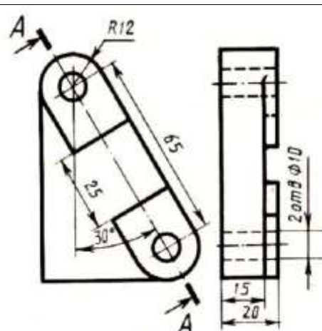
Пластина
