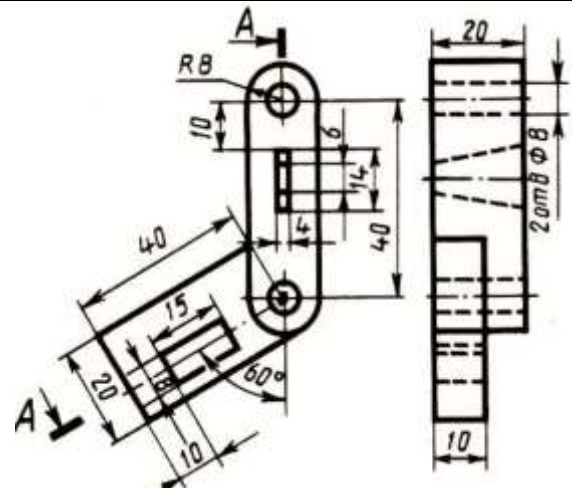
Замок
