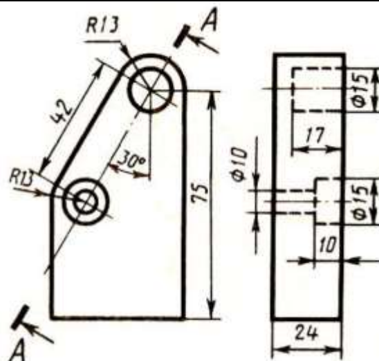
Планка
