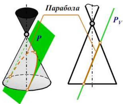
Рисунок 3 Сечение конуса плоскостью
