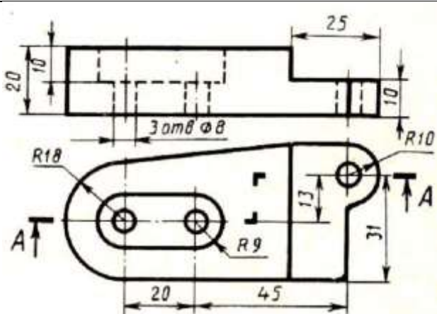
Плита
