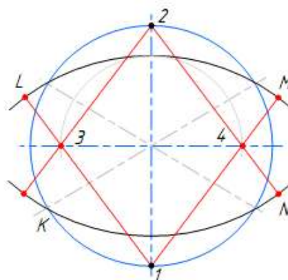
Определение точек сопряжения малых и больших дуг эллипса (точки L, M, N и K)
