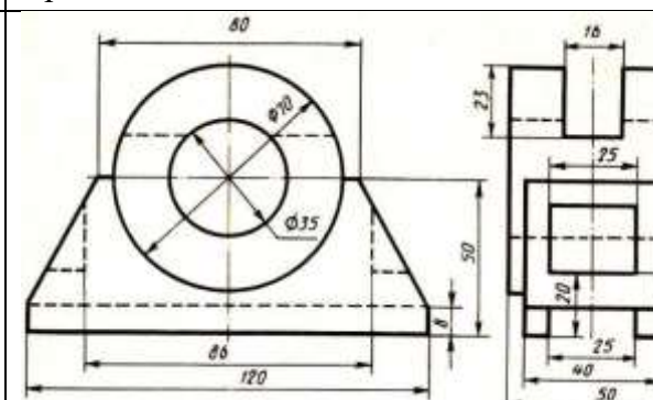
Подшипник
