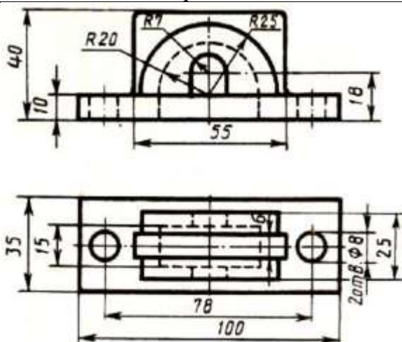
Крышка
