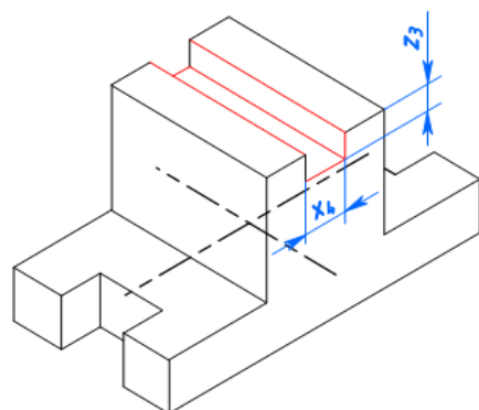
Изображение паза
