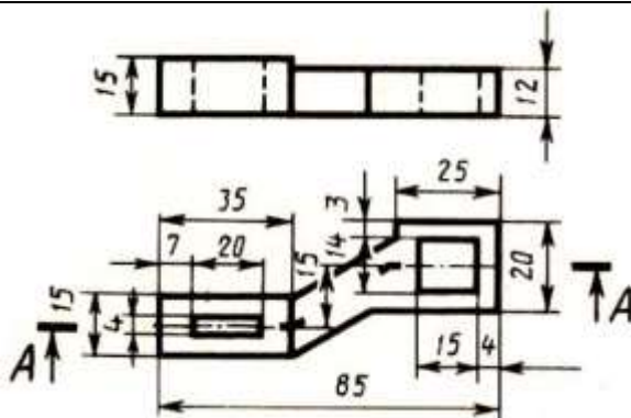
Брусок
