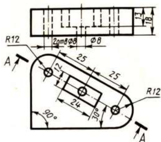
Пластина
