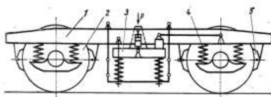
Рисунок 1 Схема тележки КВЗ-ЦНИИ 1
