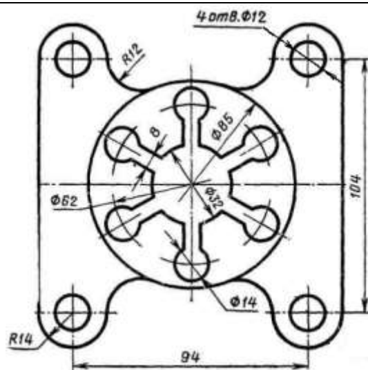
Крышка
