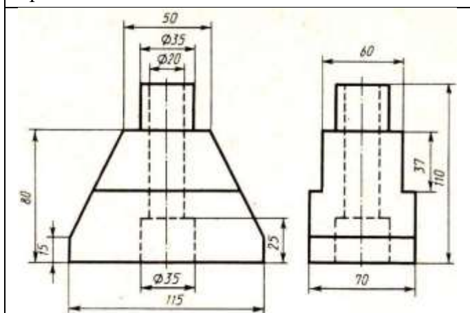
Станина
