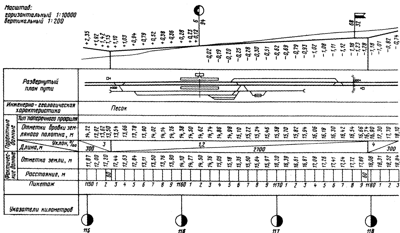
Рисунок 4 Образец выполнения продольного профиля промежуточной станции
