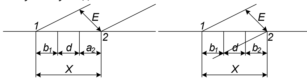
Рисунок 6 Схемы взаимного расположения двух стрелочных переводов.
