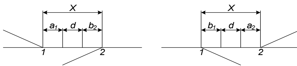
Рисунок 5 Схемы взаимного расположения стрелочных переводов при попутной укладке.
