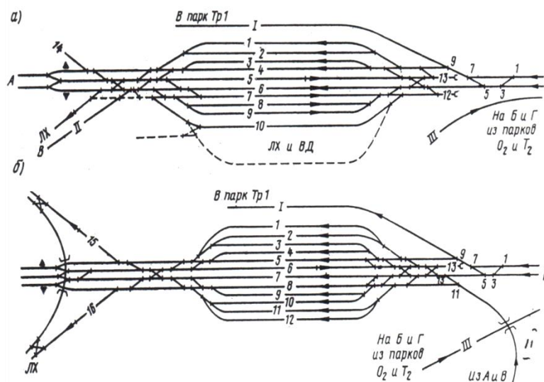
Рис 1. Схемы парка приема односторонних сортировочных станций
