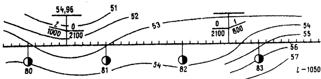
Рисунок 2 Пример продольного профиля в горизонталях
