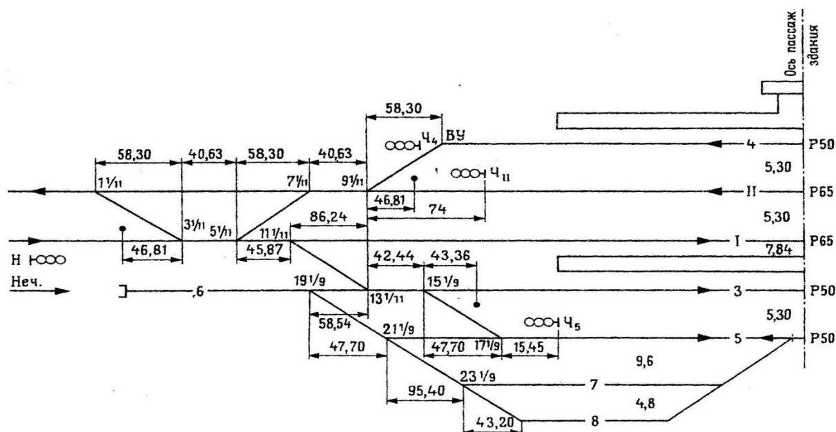
Рисунок 5 Пример установки сигналов в нечетной горловине станции
