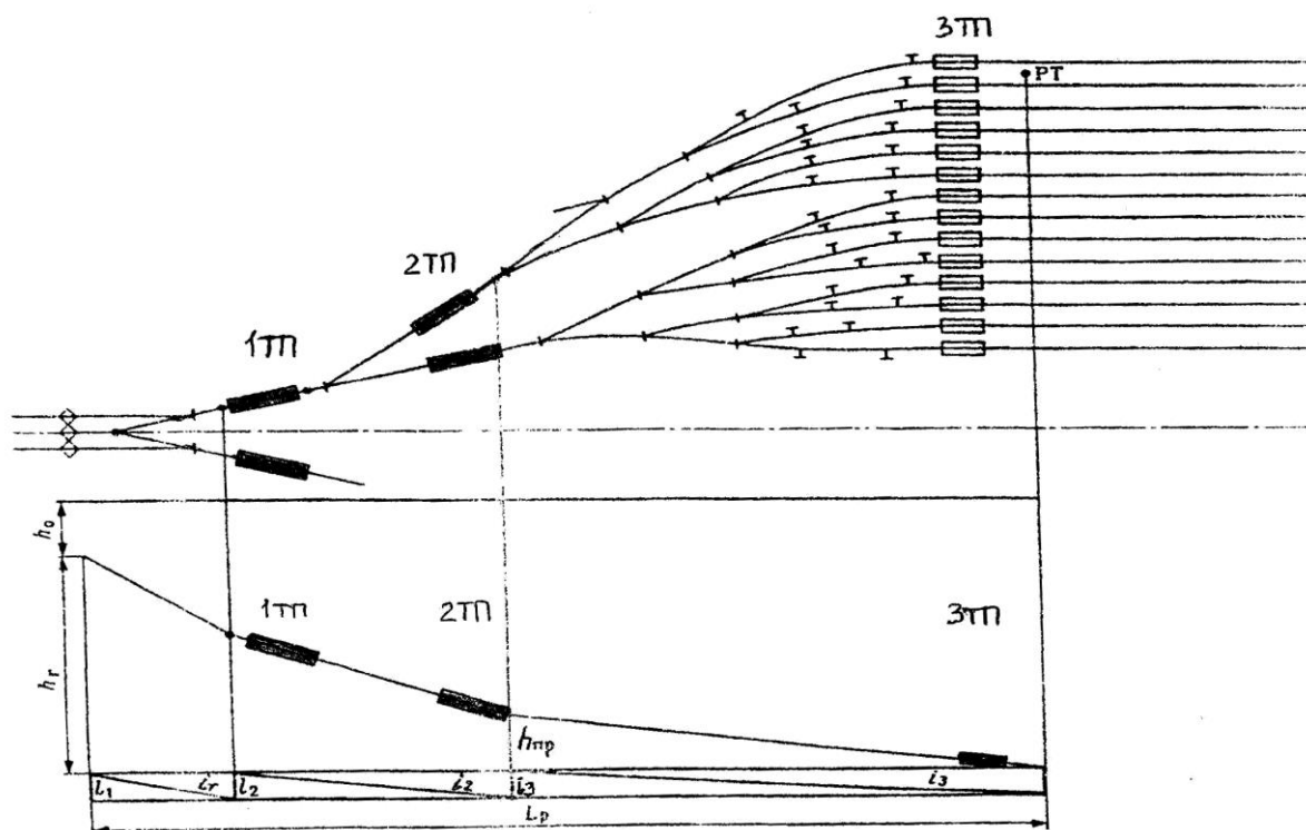
Рис. 1 План и профиль спускной части горки
