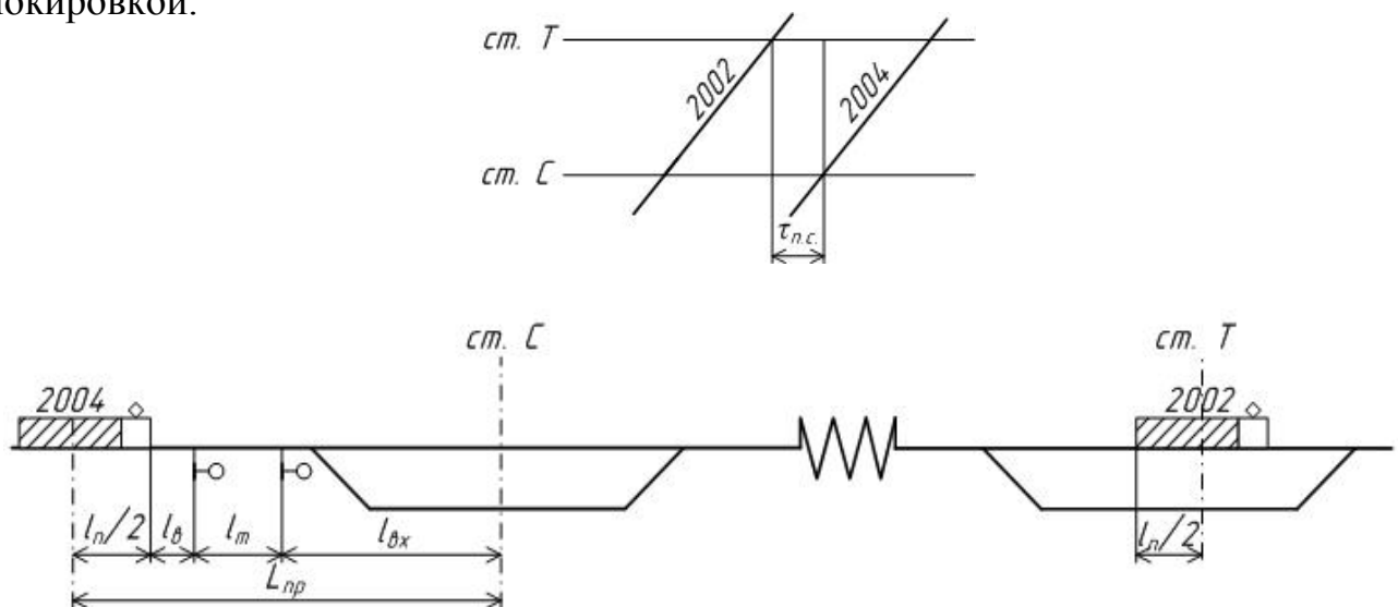
Рисунок 8 Схема расположения поездов при расчете интервала попутного следования при полуавтоматической блокировке
