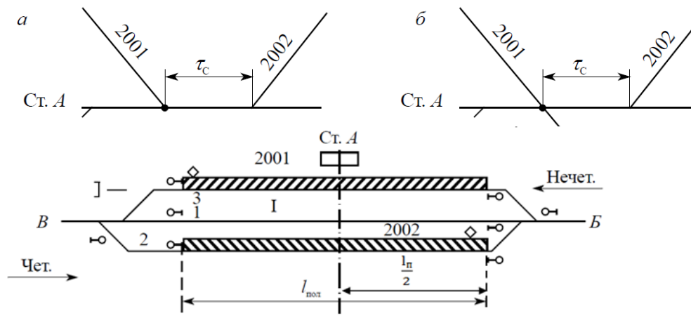
Рисунок 5 Схема расположения поездов при расчете интервала скрещения
