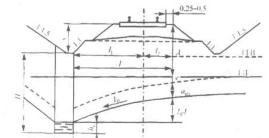
Рис. 3.1 Схема одностороннего подкюветного дренажа
